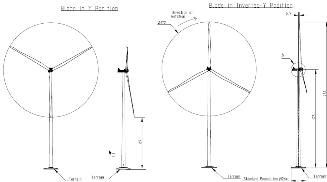
Abbildung 3: Vorder- und Seitenansicht Vestas V172 7,2 MW
