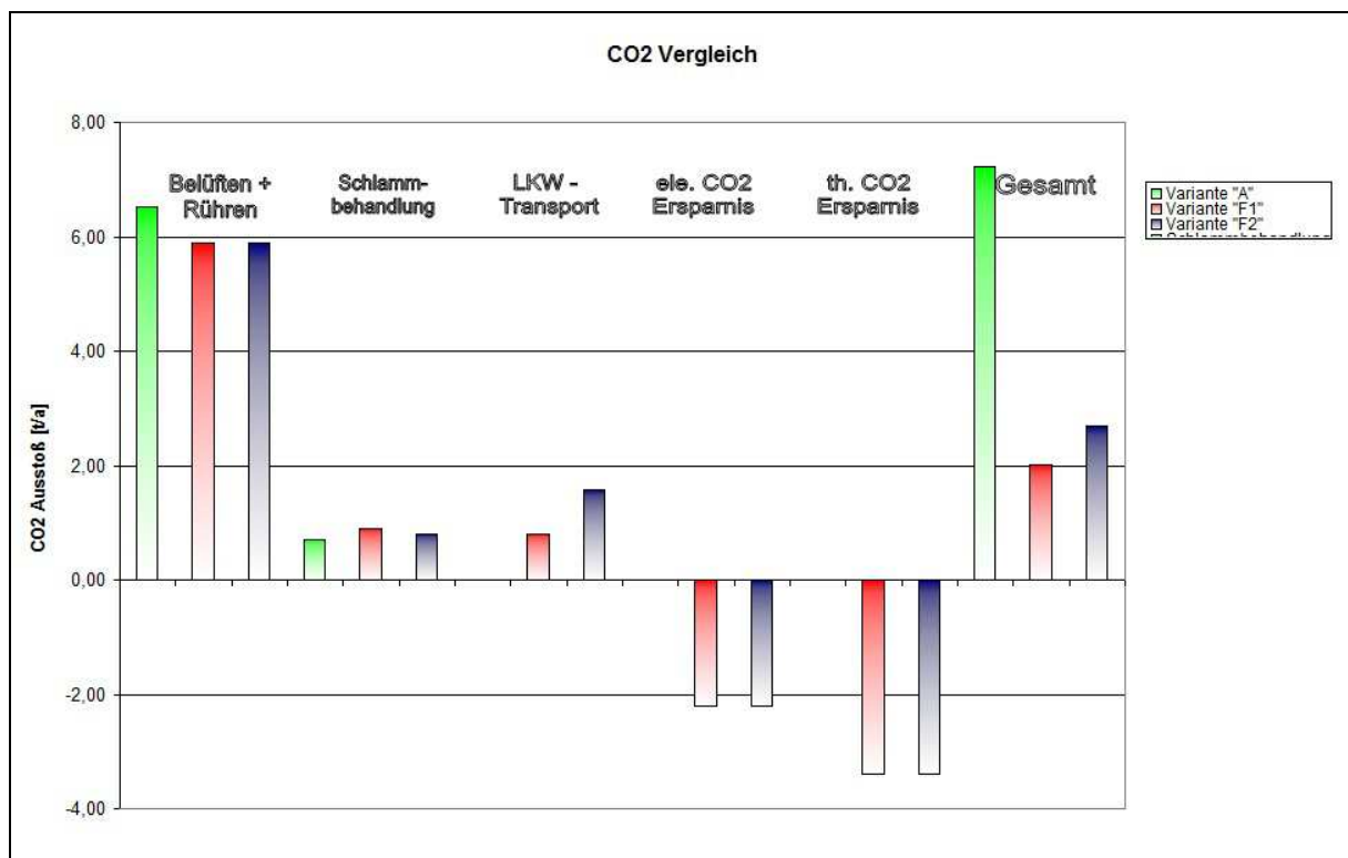
Abbildung 7: CO 2 Vergleich Beispiel 3
