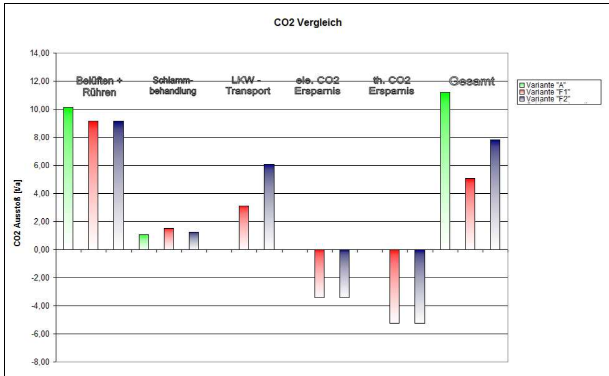
Abbildung 5:CO2 Vergleich Beispiel 2
