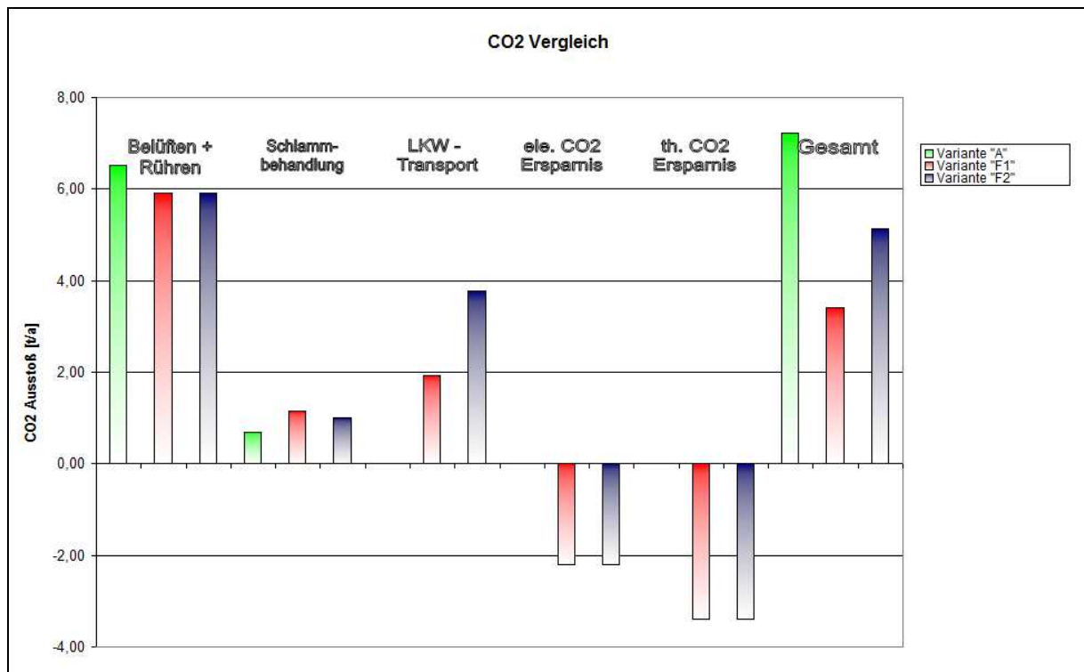
Abbildung 3:CO 2 Vergleich Beispiel 1
