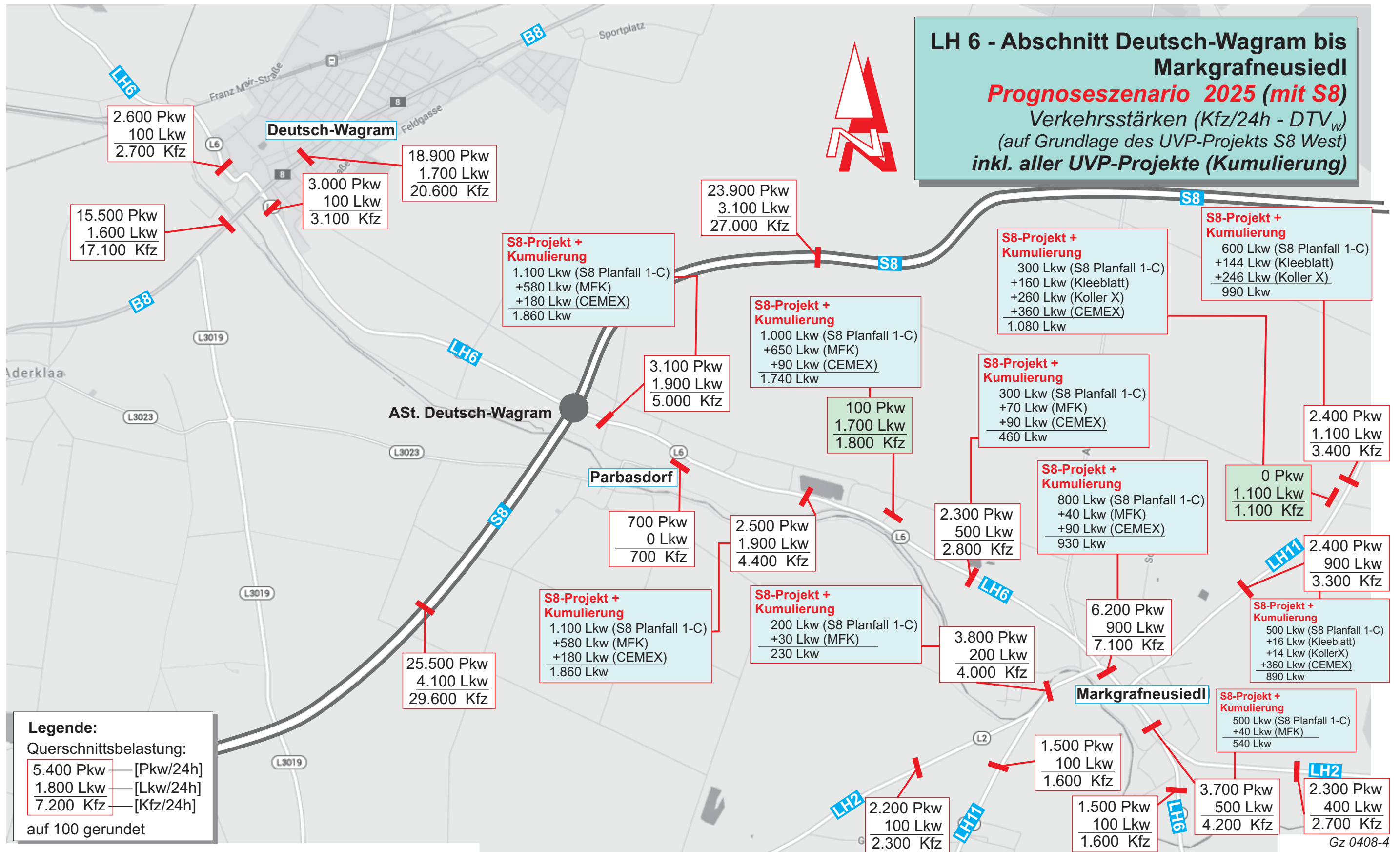
Abbildung 2.3-2: Verkehrsstärken Prognoseszenario 2025 (inkl. S 8) inkl. aller UVP-Projekte (Kumulierung)
